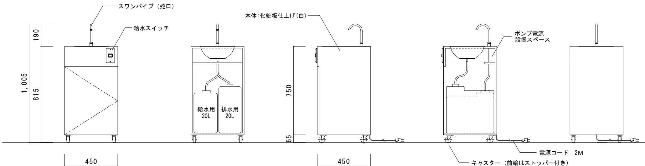
正面図
