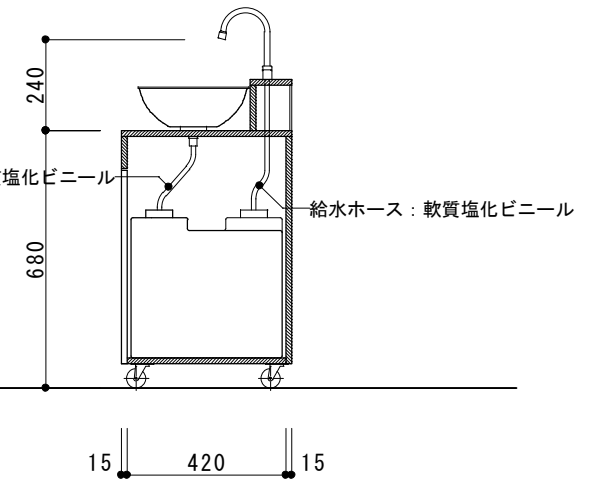
側断面図
