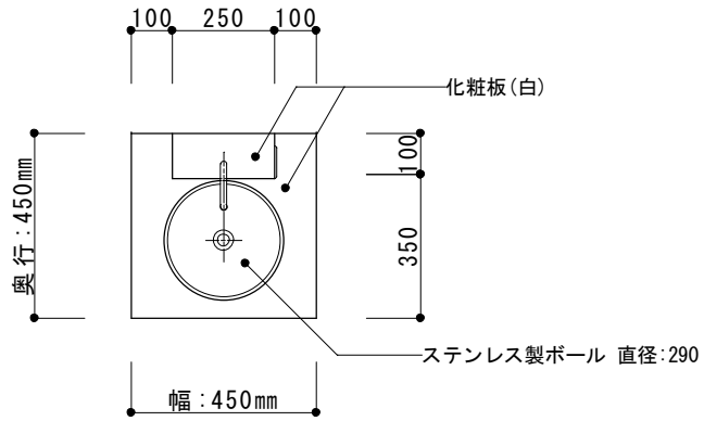
平面図
