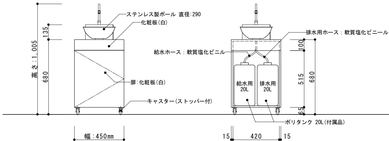
正面図
